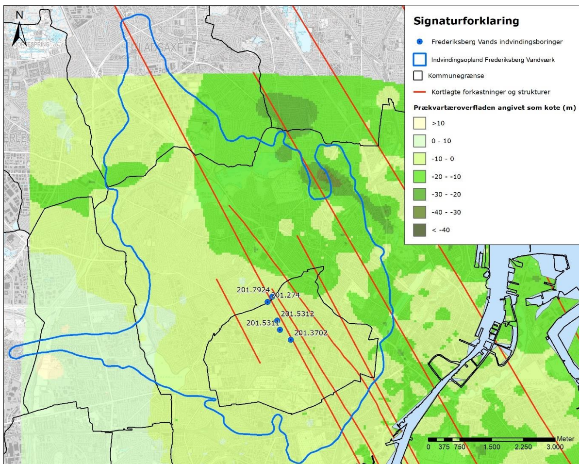
Figur 8-7: Prækvartæroverfladens højdeforhold vist sammen med kendte forkastninger og andre strukturer.
