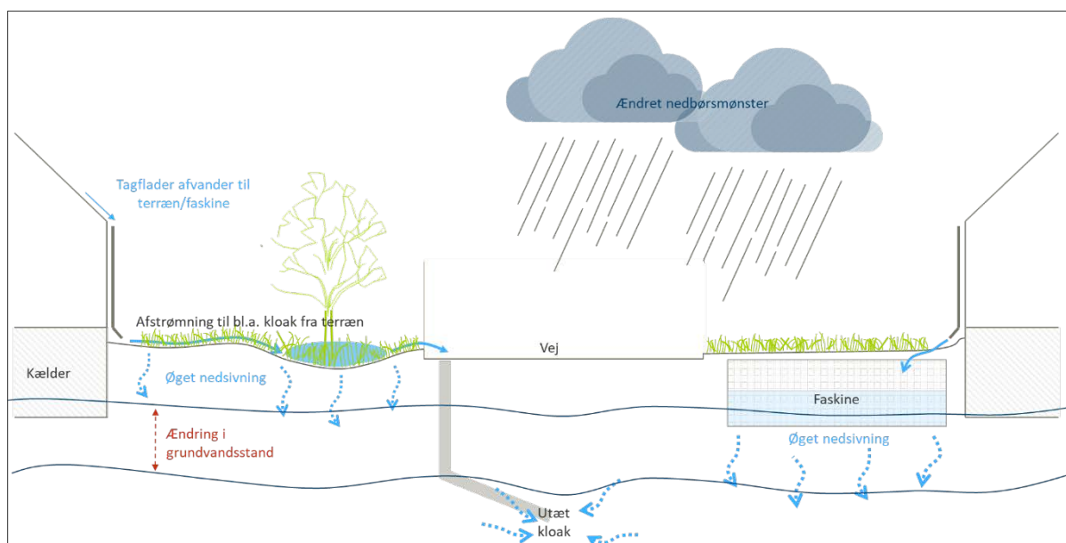
Figur 3-2: Sammenhæng mellem nedbør, grundvandsdannelse, afløbssystem mv. Øget nedbør medfører øget grundvandsdannelse. Hvis grundvandsstanden i undergrunden stiger, kan det blandt andet resultere i indsivning af grundvand i kældre og utætte kloakledninger.
