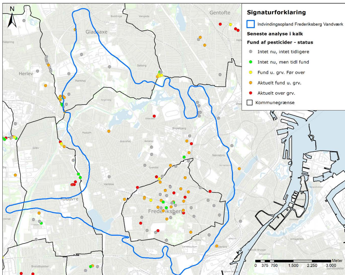
Figur 8-25: Aktuell status for indhold af pesticider i kalkmagasinet.
