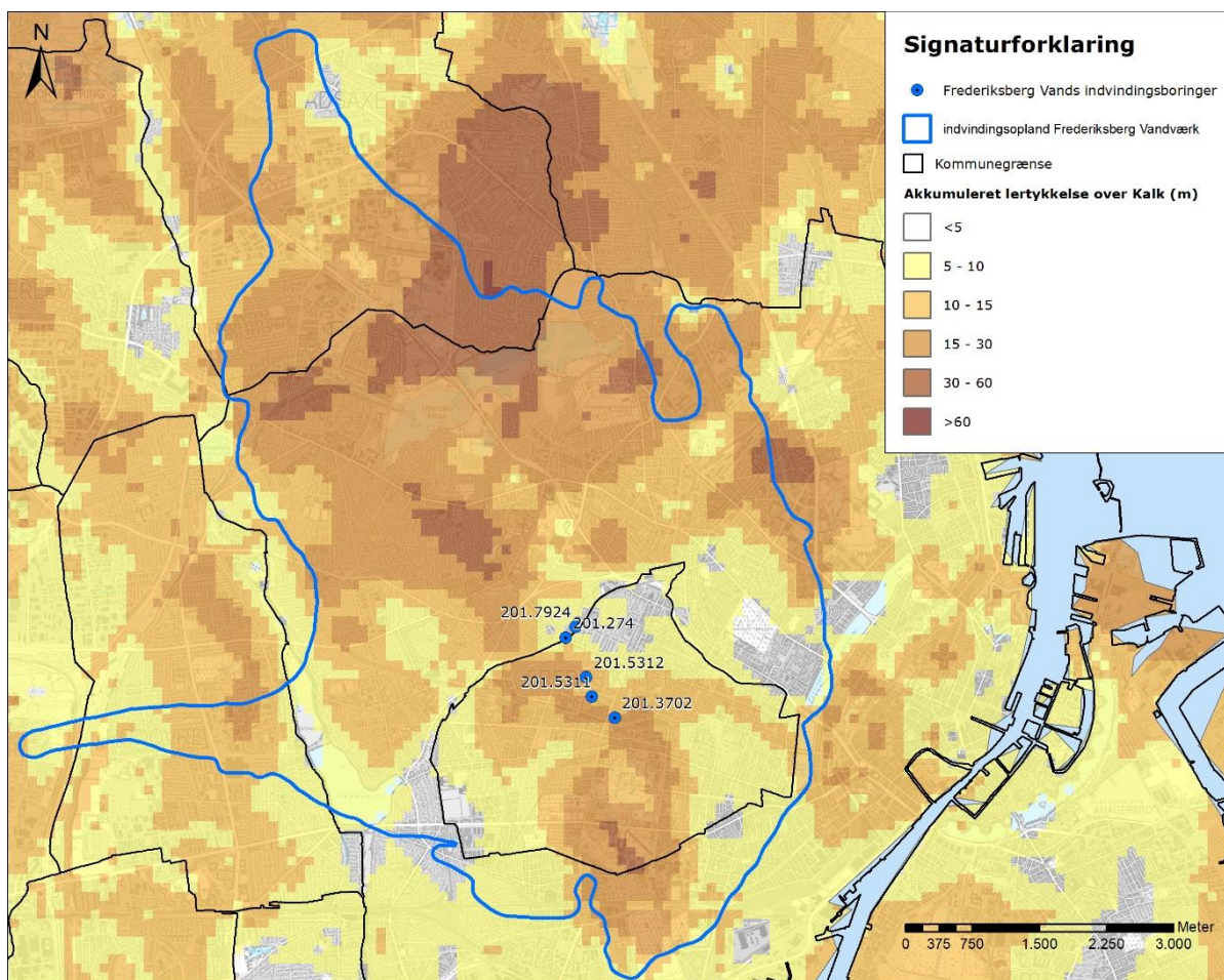
Figur 8-6: Akkumuleret leretykkelse over kalkmagasinet.
