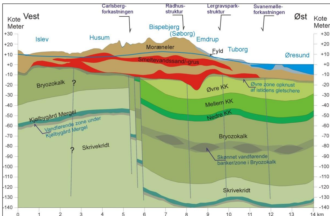
Figur 8-4: Princip for geologien i Københavnsområdet. Carlsbergforkastningen vil i nogle områder ikke have form som en trappforkastning som vist på skitsen, men mere have form, som vist på Figur 8-5.
