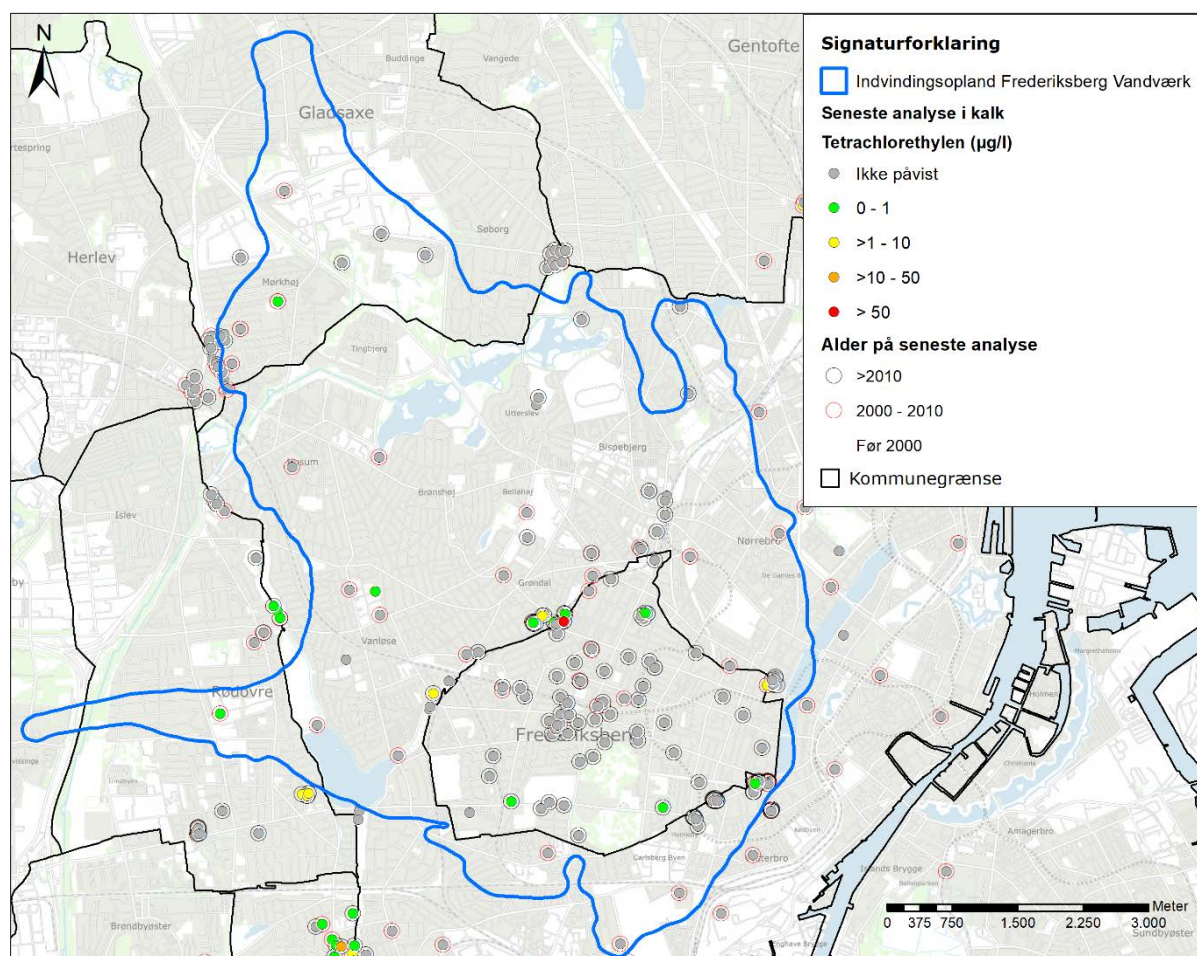
Figur 8-18: Indhold af Tetrachlorethylen (PCE) i kalkmagasinet. Kvalitetskriteriet for PCE i drikkevand er 1 µg/l.
