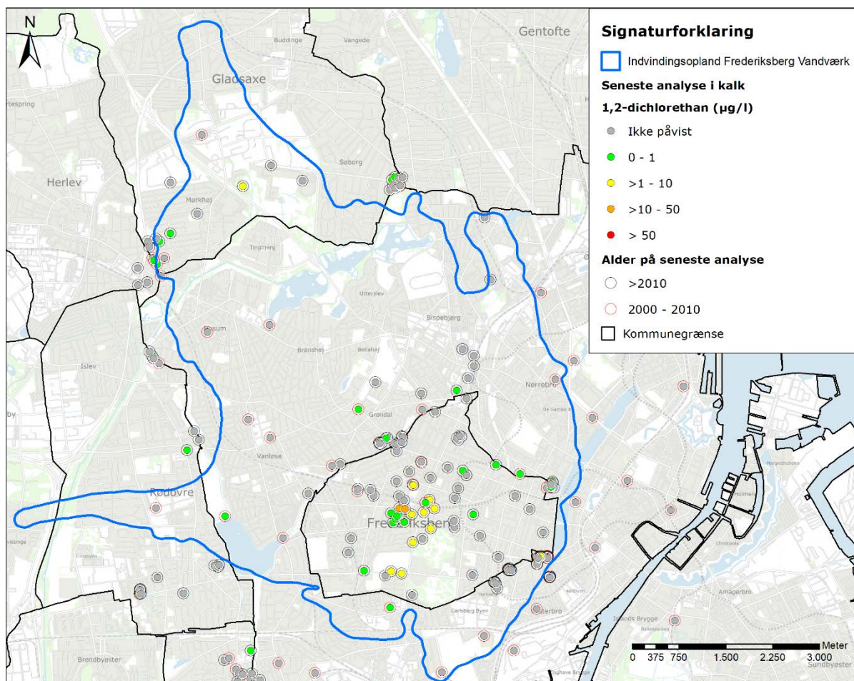
Figur 8-21: Indhold af 1,2-Dichlorethan (1,2-DCA) i kalkmagasinet. Kvalitetskriteriet for 1,2-DCA i drikkevand er 1 µg/l.
