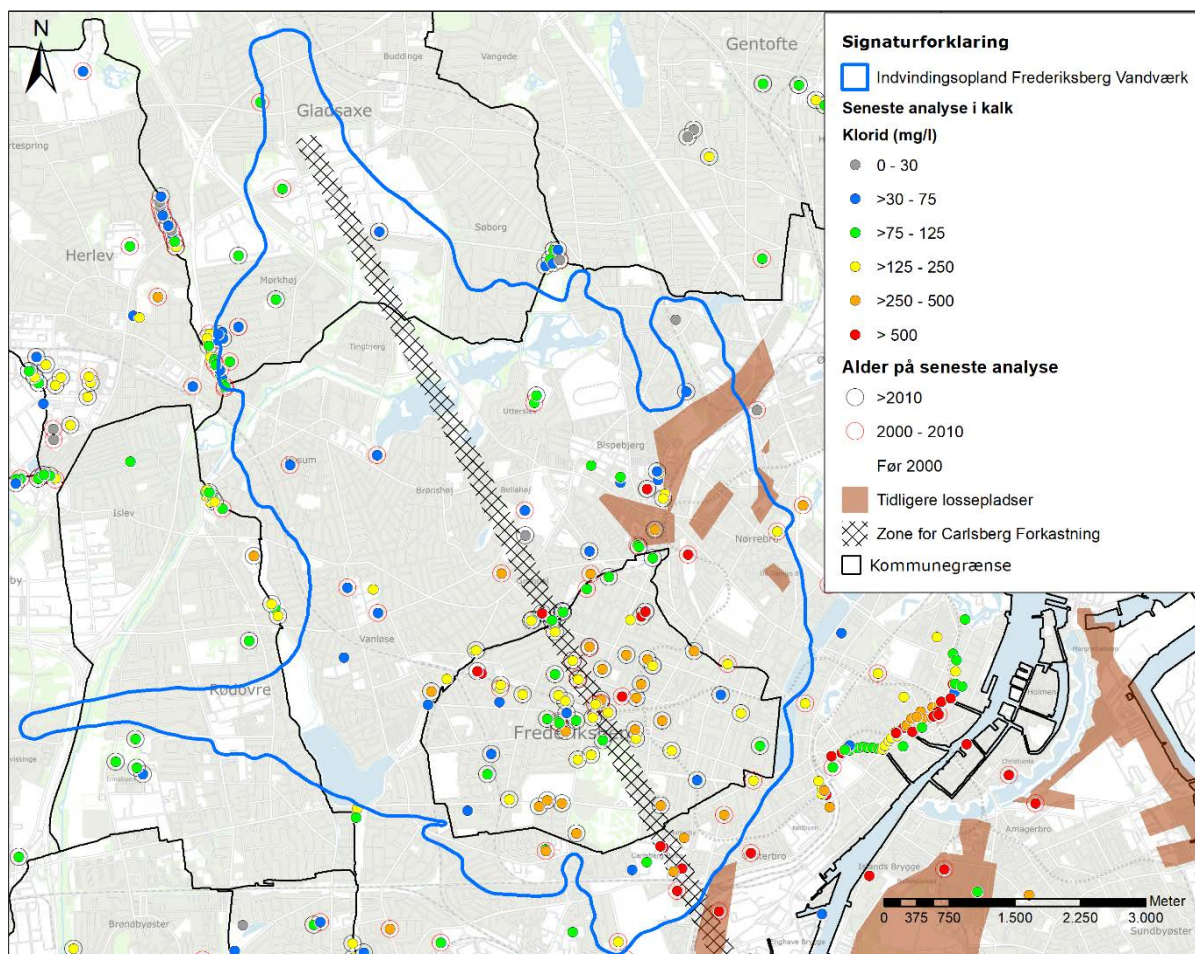
Figur 8-13: Indhold af klorid i kalkmagasinet vist sammen med tidligere lossepladser og beliggenheden af Carlsbergforkastningen. Kvalitetskriteriet for klorid i drikkevand er 250 mg/l
