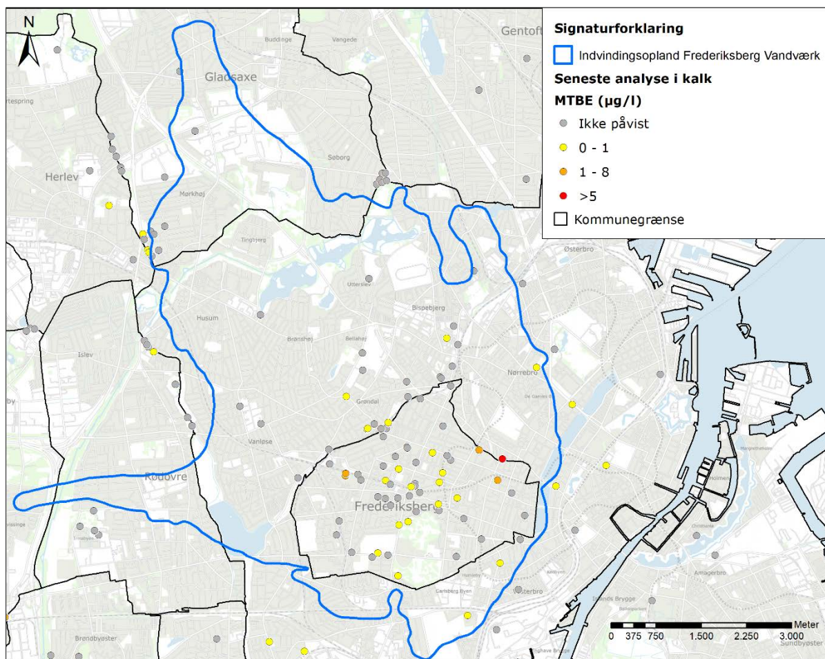
Figur 8-23: Indhold af MTBE i kalkmagasinet. Kvalitetskriteriet for MTBE i drikkevand er 5 µg/l.
