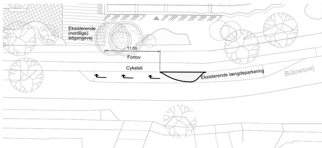
Figur 2: Nordlig ind- og udkørsel. Illustration fra den trafikale analyse, tegning K11_N1101, rev. C dateret 26.04.2019, MOE | Tetraplan
